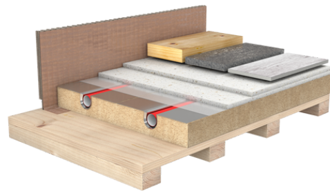
Exemplarischer Bodenaufbau
