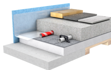
Exemplarischer Bodenaufbau
