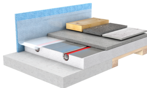
Exemplarischer Bodenaufbau
