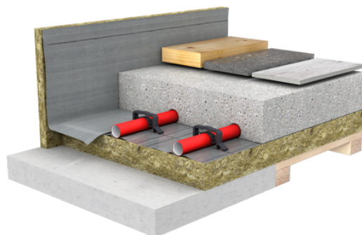
Exemplarischer Bodenaufbau
