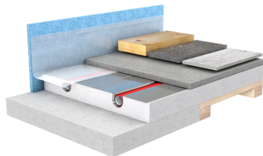
Exemplarischer Bodenaufbau
