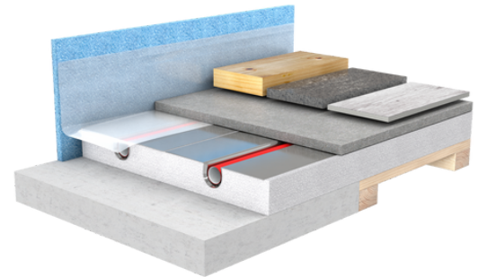
Exemplarischer Bodenaufbau
