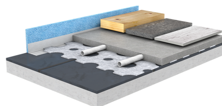
Exemplarischer Bodenaufbau
