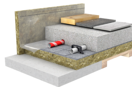
Exemplarischer Bodenaufbau
