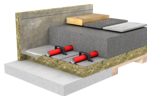
Exemplarischer Bodenaufbau
