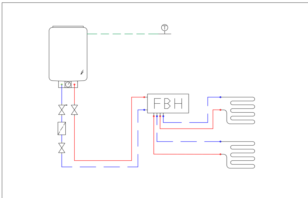
Anschlussschema des Heizkessels an eine Flächenheizungsanlage
