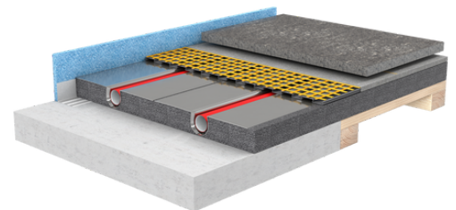
Exemplarischer Bodenaufbau
