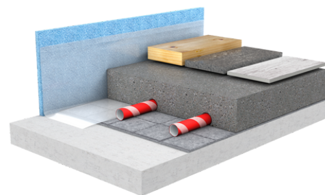
Exemplarischer Bodenaufbau
