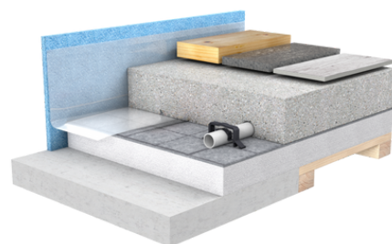
Exemplarischer Bodenaufbau
