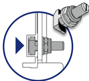
Giunzione del fermapiede
