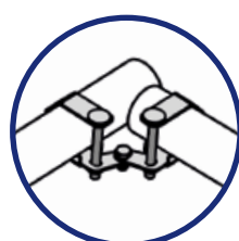
Giunto e giunzione angolare con attacco al terminale del corrimano / corrente intermedio
