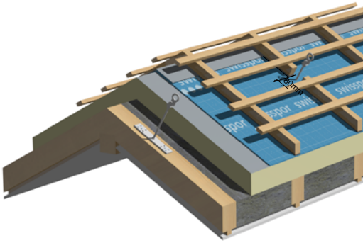
Seilsicherungssystem
